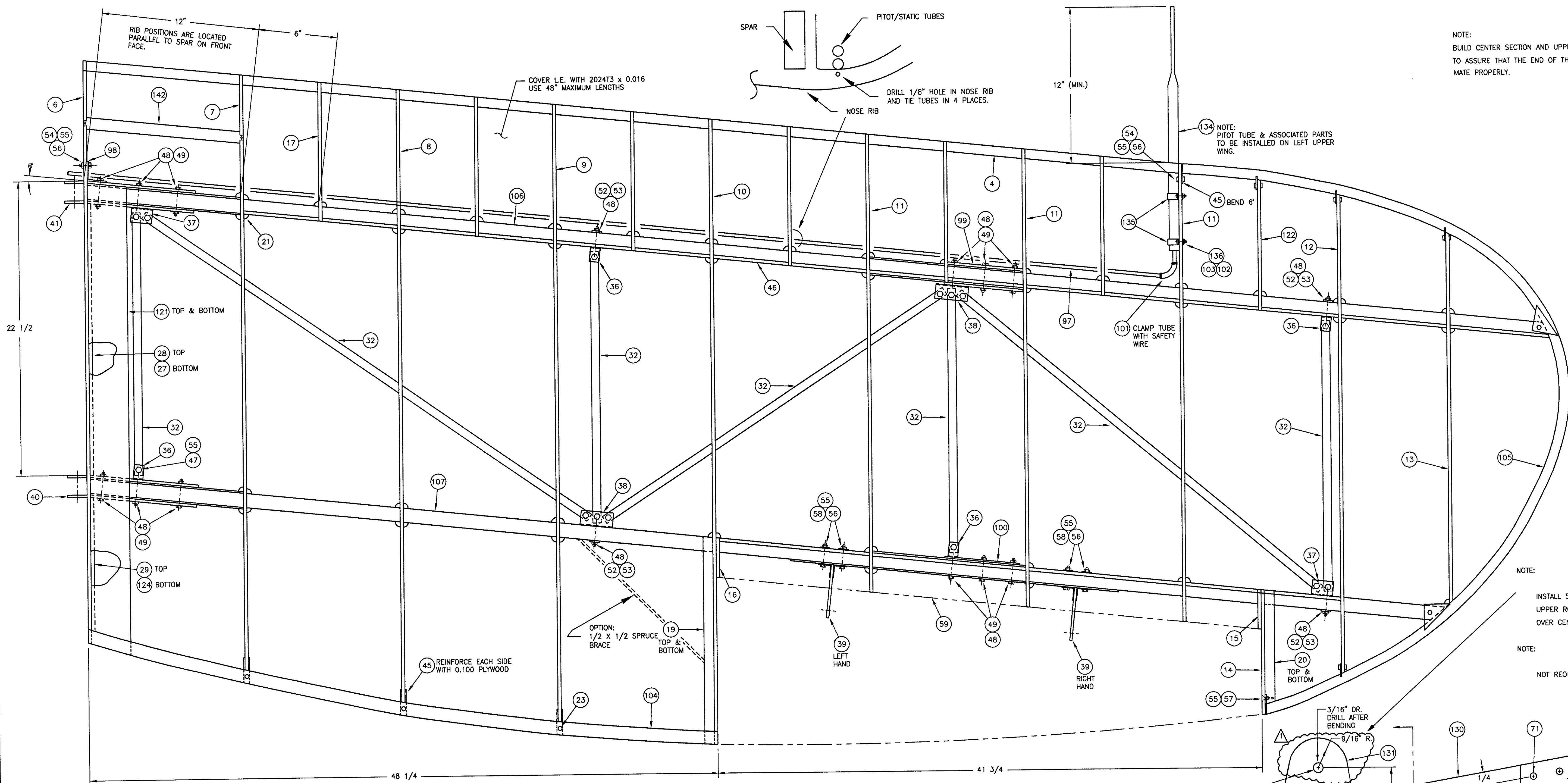
UPPER WING ASSEMBLY SCALE: 3"=1'-0"
